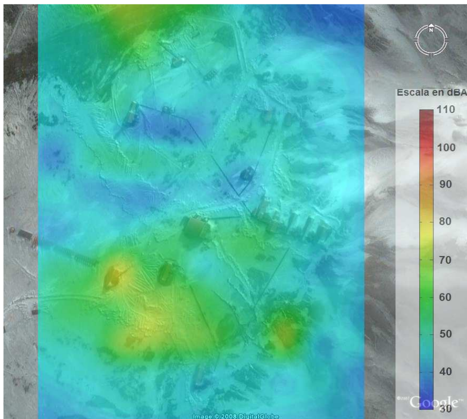
Figura 13. Mapa de ruido de la Base con Hércules C-130 en pista.
