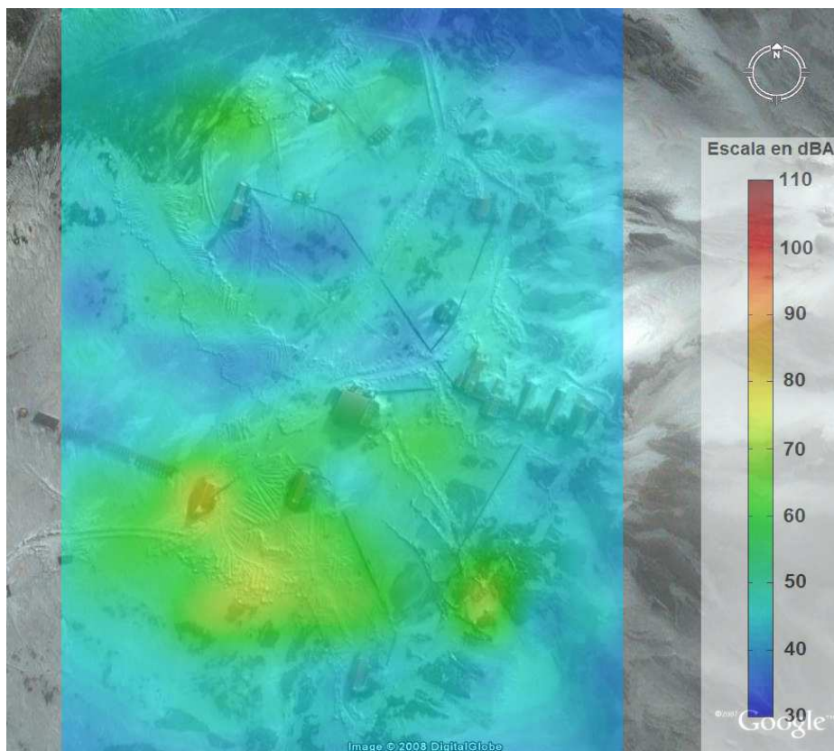
Figura 11. Mapa de ruido de la base con actividad normal.
