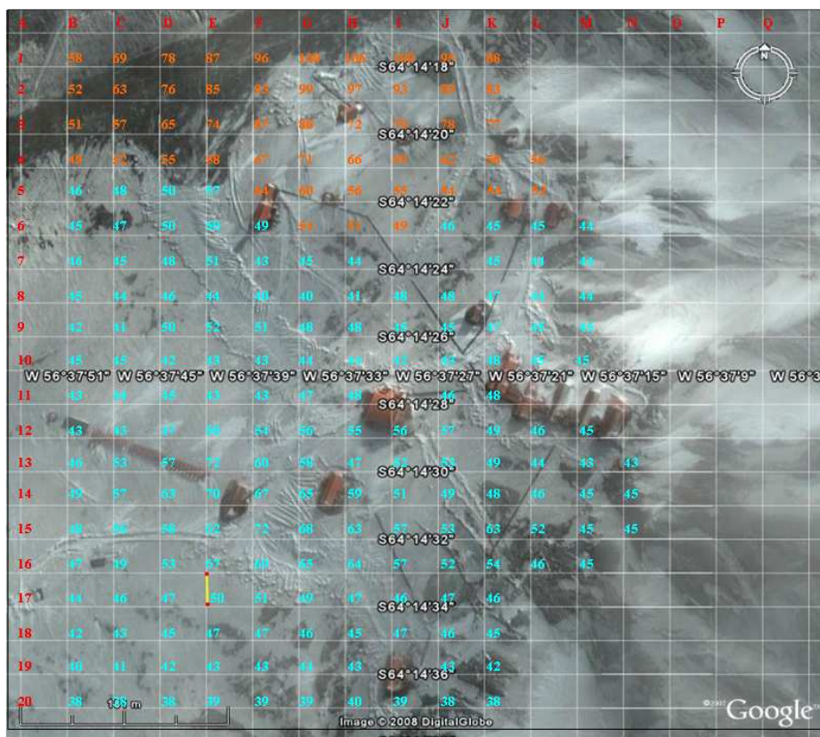
Figura 18. Grilla con niveles sonoros en dBA.
