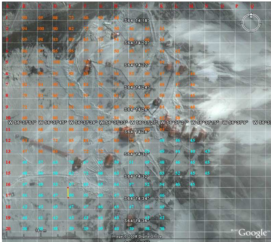
Figura 20. grilla con niveles sonoros en dBA.
