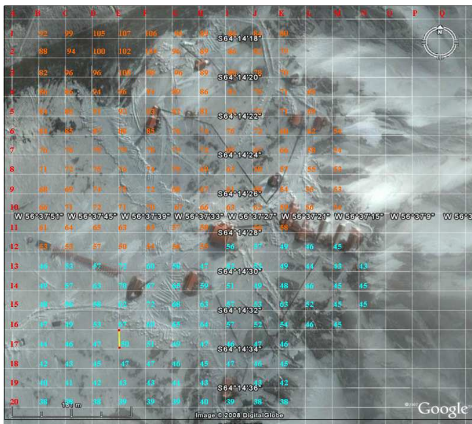
Figura 14. Grilla con niveles sonoros en dBA.
