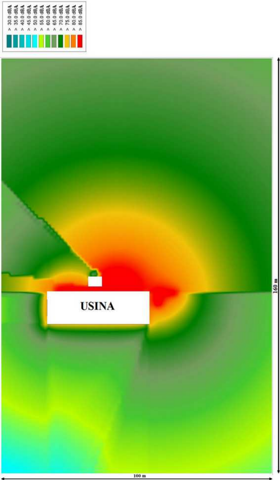
Figura 7. Mapa de ruido alrededor de la usina.
