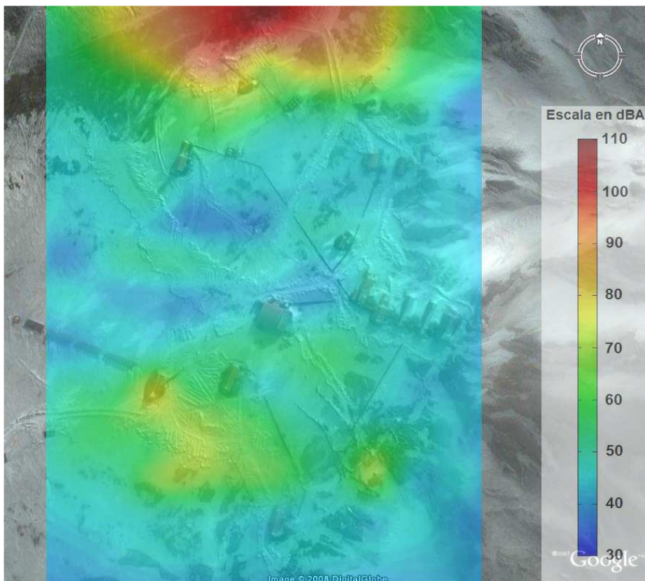
Figura 19. Mapa de ruido con Bell 212 en aprovisionamiento y traslado de personal.
