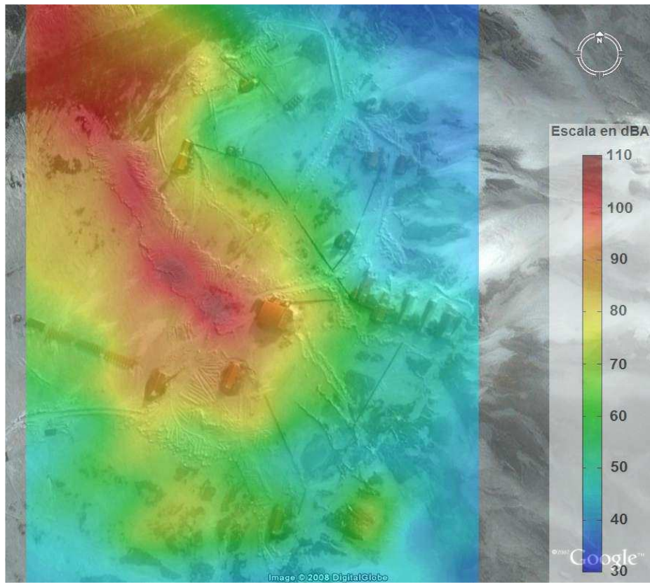
Figura 21. Mapa de ruido con Twin Otter realizando entrenamiento y traslado a pista.
