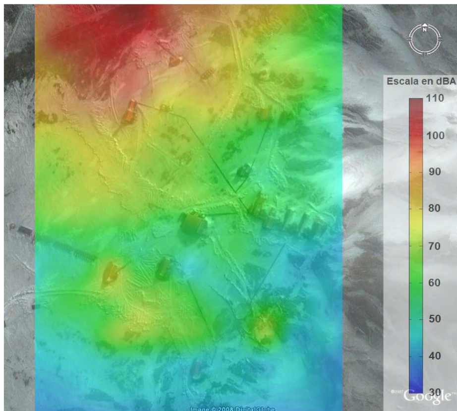
Figura 15. Mapa de ruido de la Base con Hércules C-130 en puesta en marcha y carreteo.
