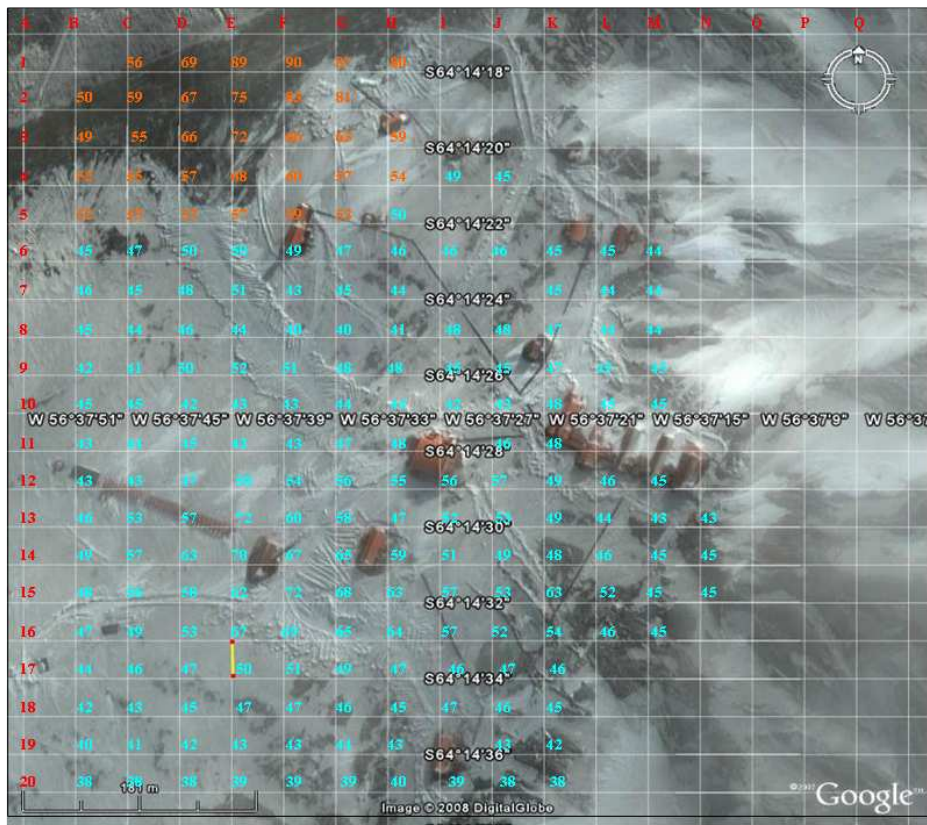
Figura 12. Grilla con niveles sonoros en dBA.
