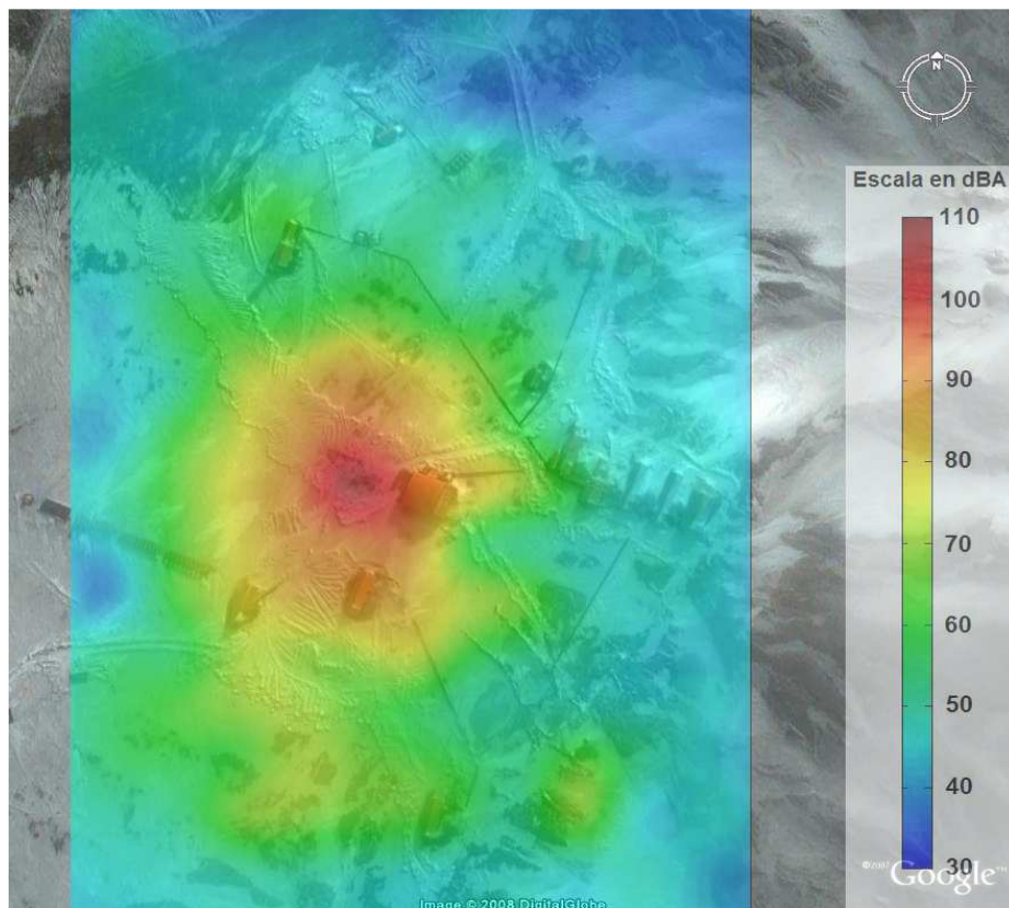
Figura 17. Mapa de ruido con helicópteros Bell 212 en check lists y entrenamientos.
