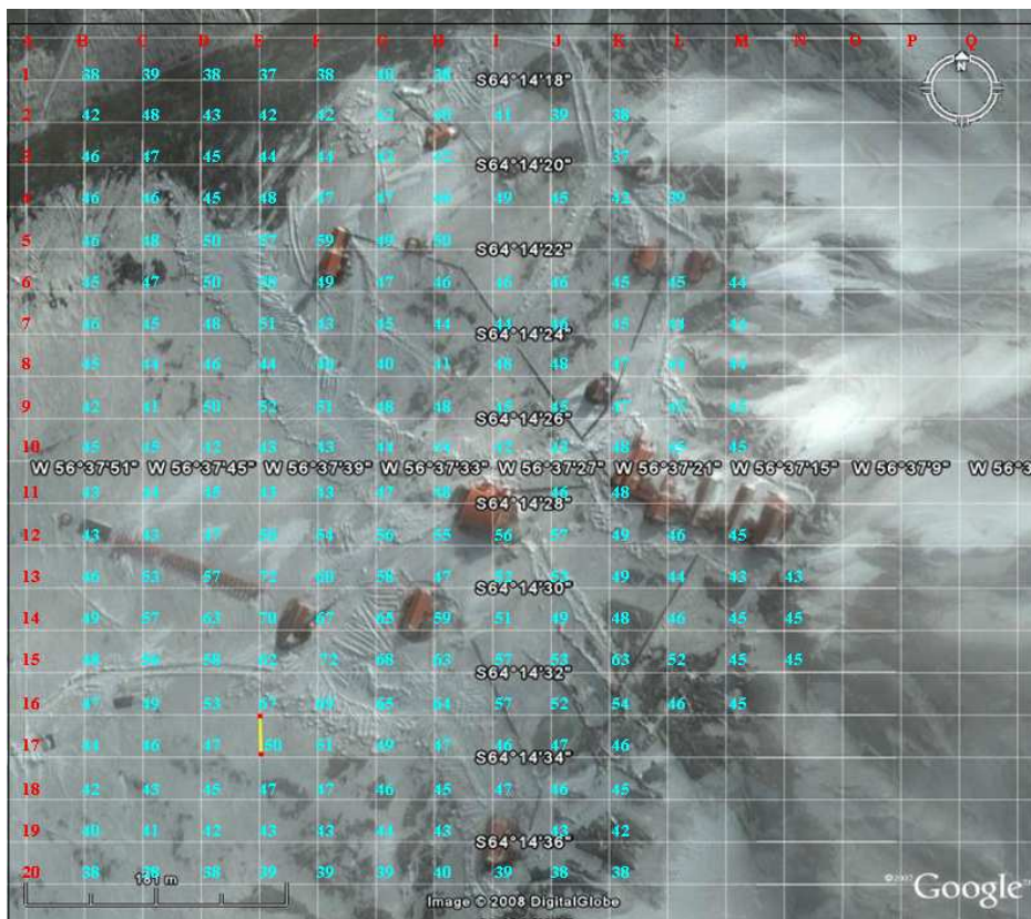
Figura 10. Grilla con coordenadas y niveles sonoros en dBA .
