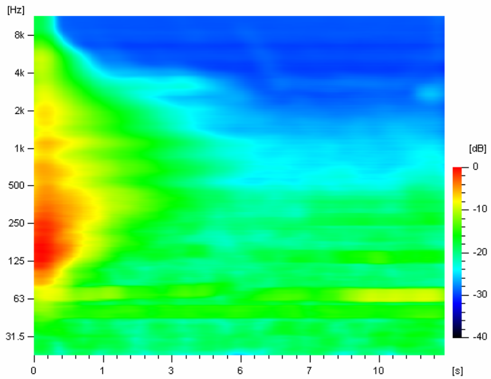
Figura 13: SUM Colegio Dr. Antonio Nores. FSO_1—M_3
