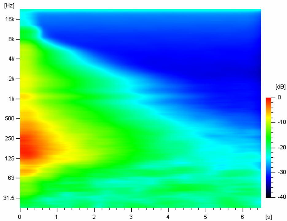
Figura 12: Parroquia Sagrado Corazón de Jesús. FSO_1-M_2
